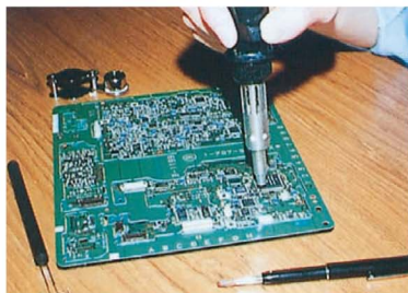
ICの取り付け
